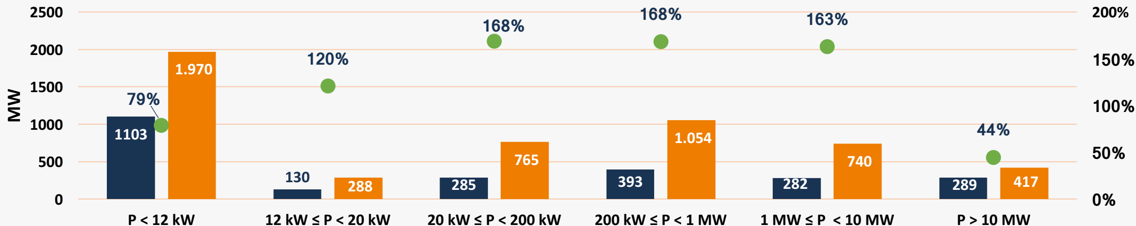
Potenza connessa per classe di potenza (asse sx) e variazione % 2023/22 (asse dx)
