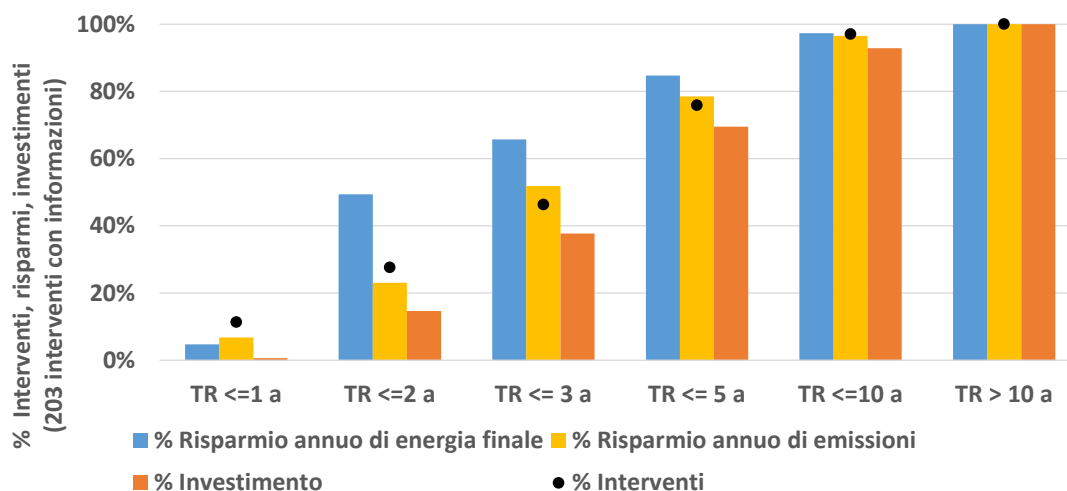
Figura 4-46. Distribuzione cumulata di risparmi di energia finale, risparmi di emissioni, investimenti e interventi per classe di tempo di ritorno
