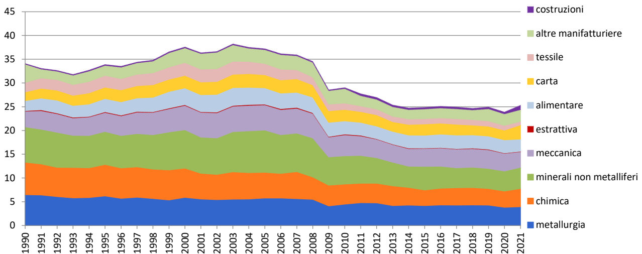
Figura 2-11. Consumo energetico finale nei settori industriali in Italia. Dettaglio per settori di attività economica, anni 1990-2021 (Mtep)
