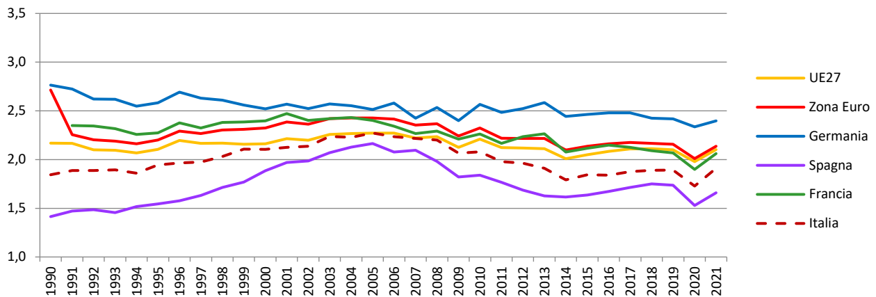
Figura 2-8. Consumi finali di energia per abitante nelle maggiori economie UE27, anni 1990-2021 (tep/abitante)
