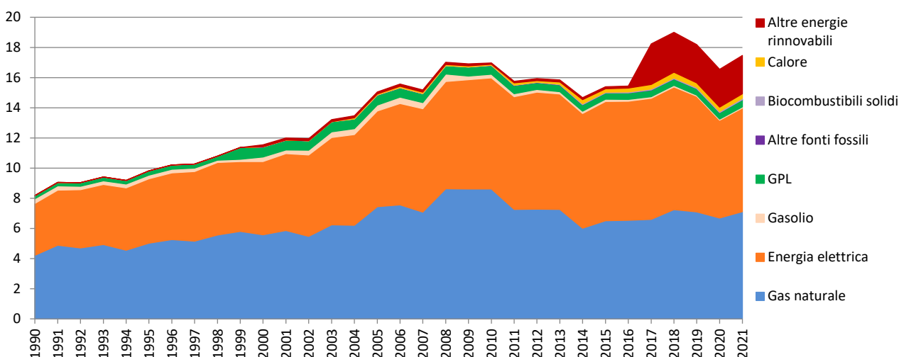
Figura 2-15. Consumo energetico nel settore servizi. Dettaglio per fonte energetica, anni 1990-2021 (Mtep)
