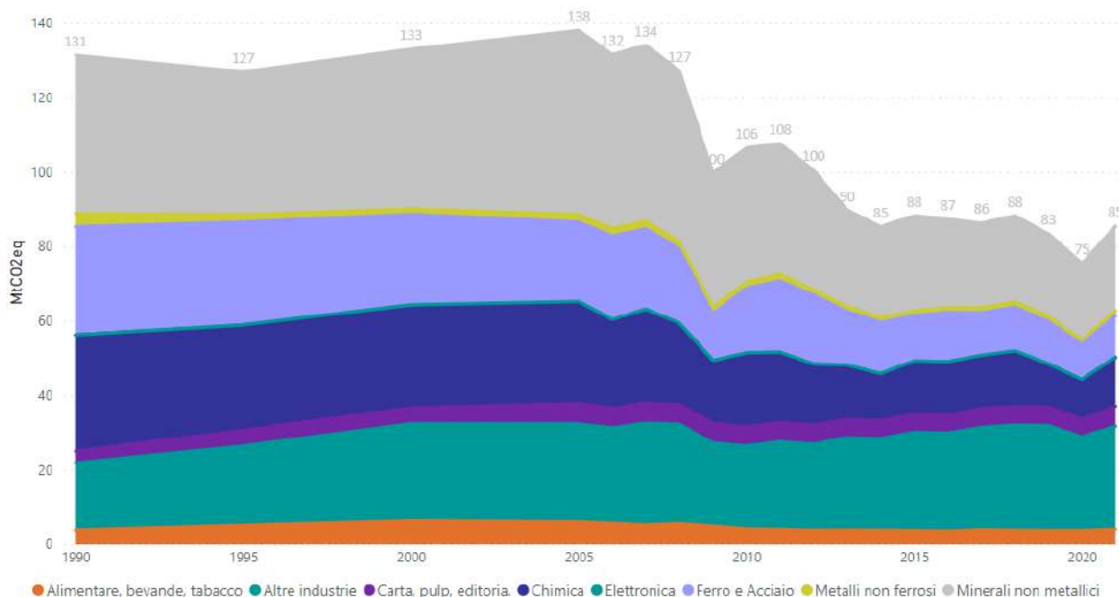
Figura 29 – Andamento delle emissioni del settore industriale (MtCO 2 eq)
